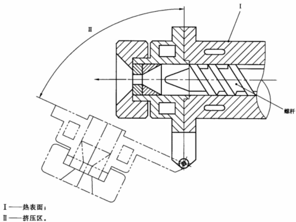
图 14 橡胶挤出机单机头主要危险区示例
