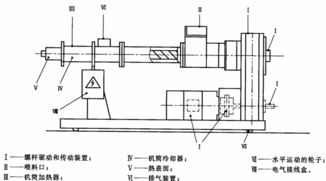
图 2 橡胶挤出机主要危险区示例
