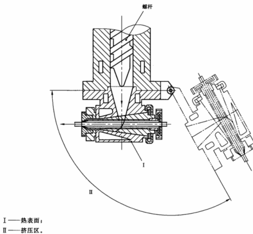
图 15 橡胶和塑料挤出机直角机头主要危险区示例
