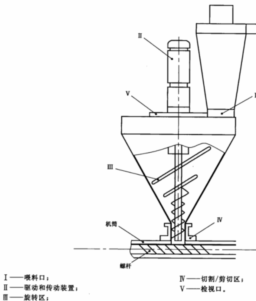
图 3 垂直填塞式喂料系统主要危险区示例
