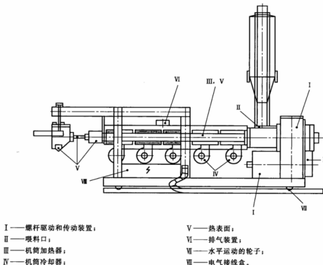
图 1 塑料挤出机主要危险区示例
