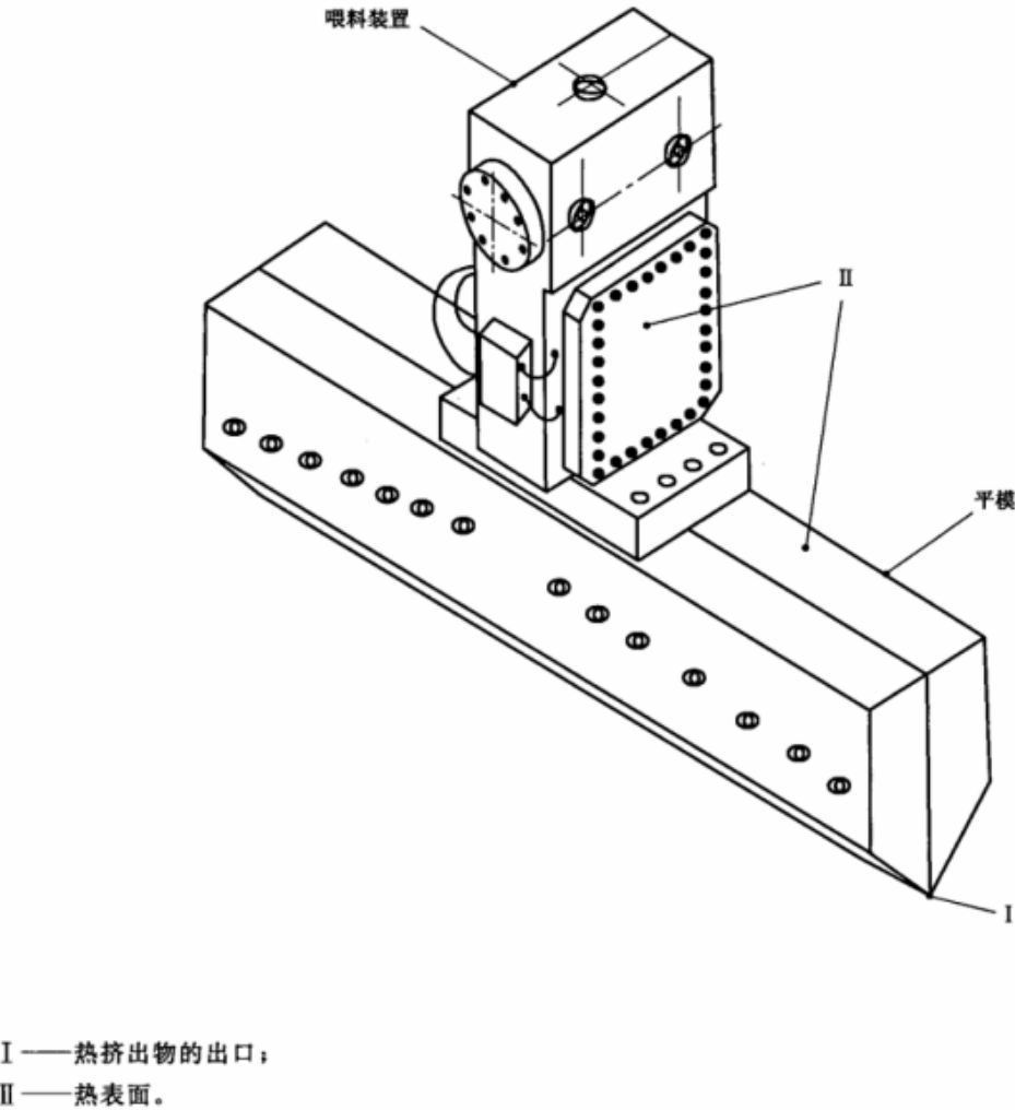
图 12 生产塑料薄膜的平模机头主要危险区示例
